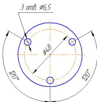
Рис.2 Разметка отверстий.
